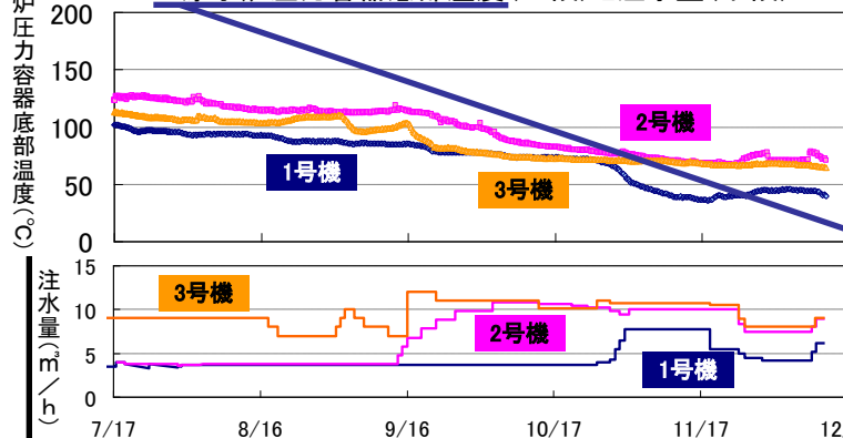
原子炉圧力容器底部温度(上段)と注水量(下段)
